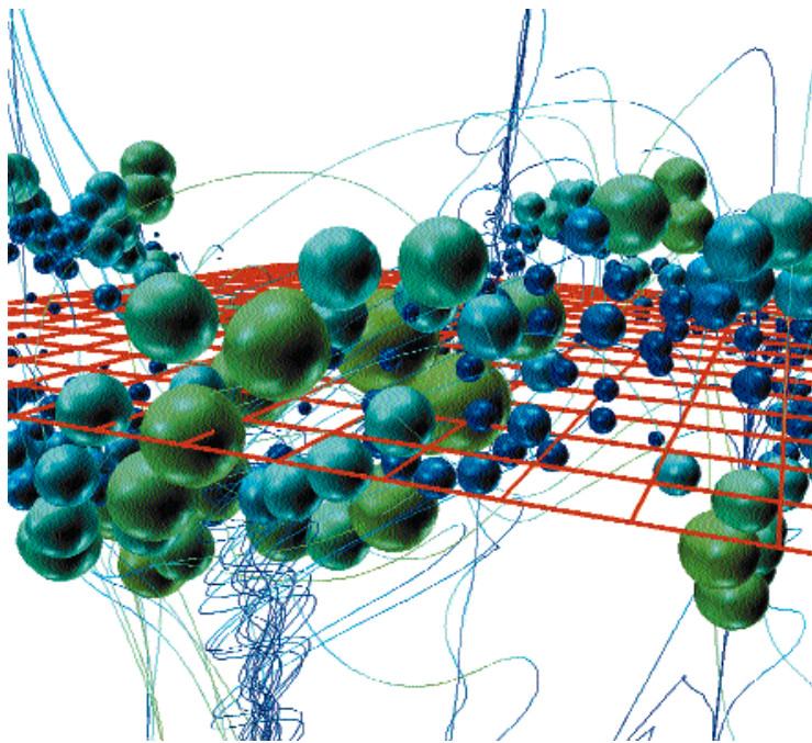
Structures d'écoulement turbulent Copyright : Anthony RANORIAMAMPINANINA, IRPHE Marseille
